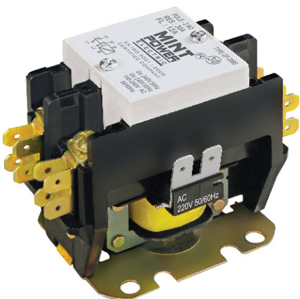
DP-2 POLE
